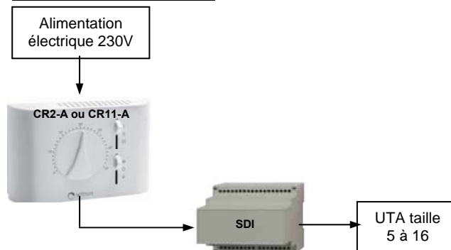
Raccordement taille 5 à 16
